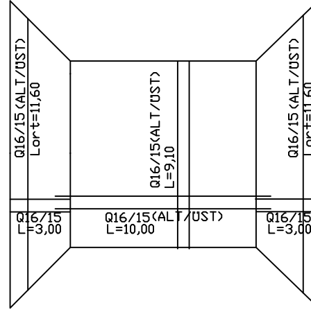
RADYE DONATI DETAYI
