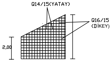
RİCAT DONATI DETAYI
