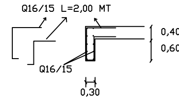
PARAFİ DONATI DETAYI
